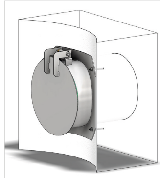
■ GW-RDD S: Rückstauklappe zum Einbau in einen Rundschaft / GW-RDD S: flap valve for installation into a round chamber
