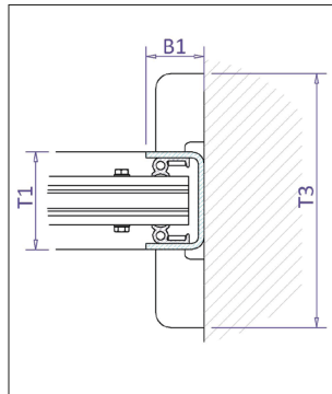
▪ Typ 2 - IDR / type 2 - IDR
