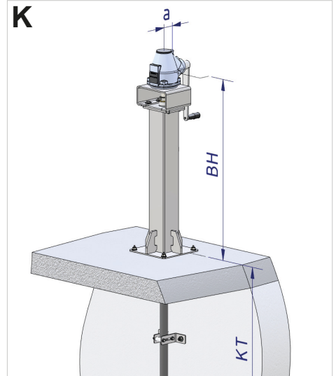
▪ Antrieb auf gerader Flursäule mittels Kegelradgetriebe und Handkurbel / drive mounted on straight headstock with bevel gearbox and crank handle
