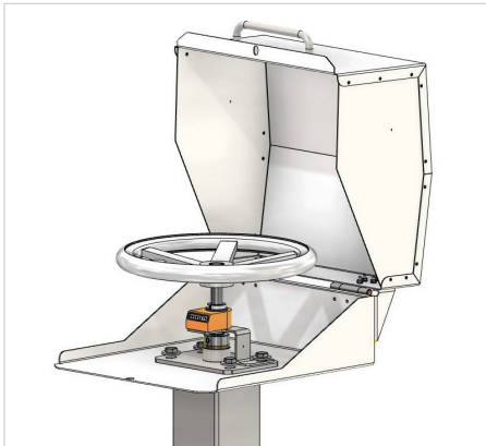
▪ Abdeckhaube für Handrad mit Stellungsanzeige / cover for hand wheel with position indicator
