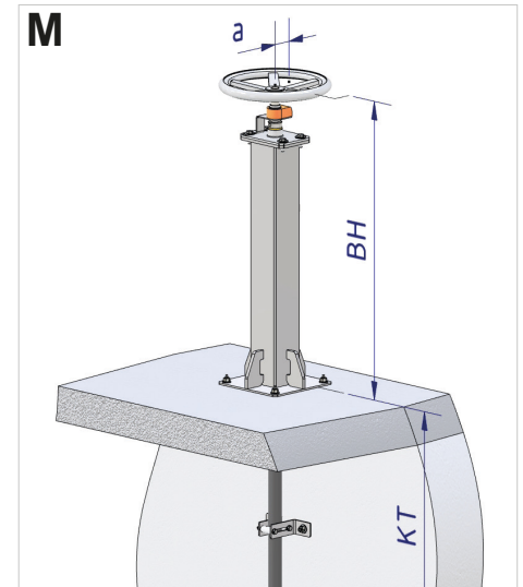
▪ Antrieb auf gerader Flursäule mittels Handrad und Stellungsanzeige / drive mounted on straight headstock with position indicator and hand wheel
