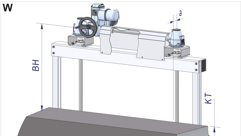
▪ Antrieb 2-spindelig auf Traverse mittels Kegelradgetrieben und E-Antrieb / 2-spindle drive mounted on crossbar with bevel gearboxes and electric actuator
